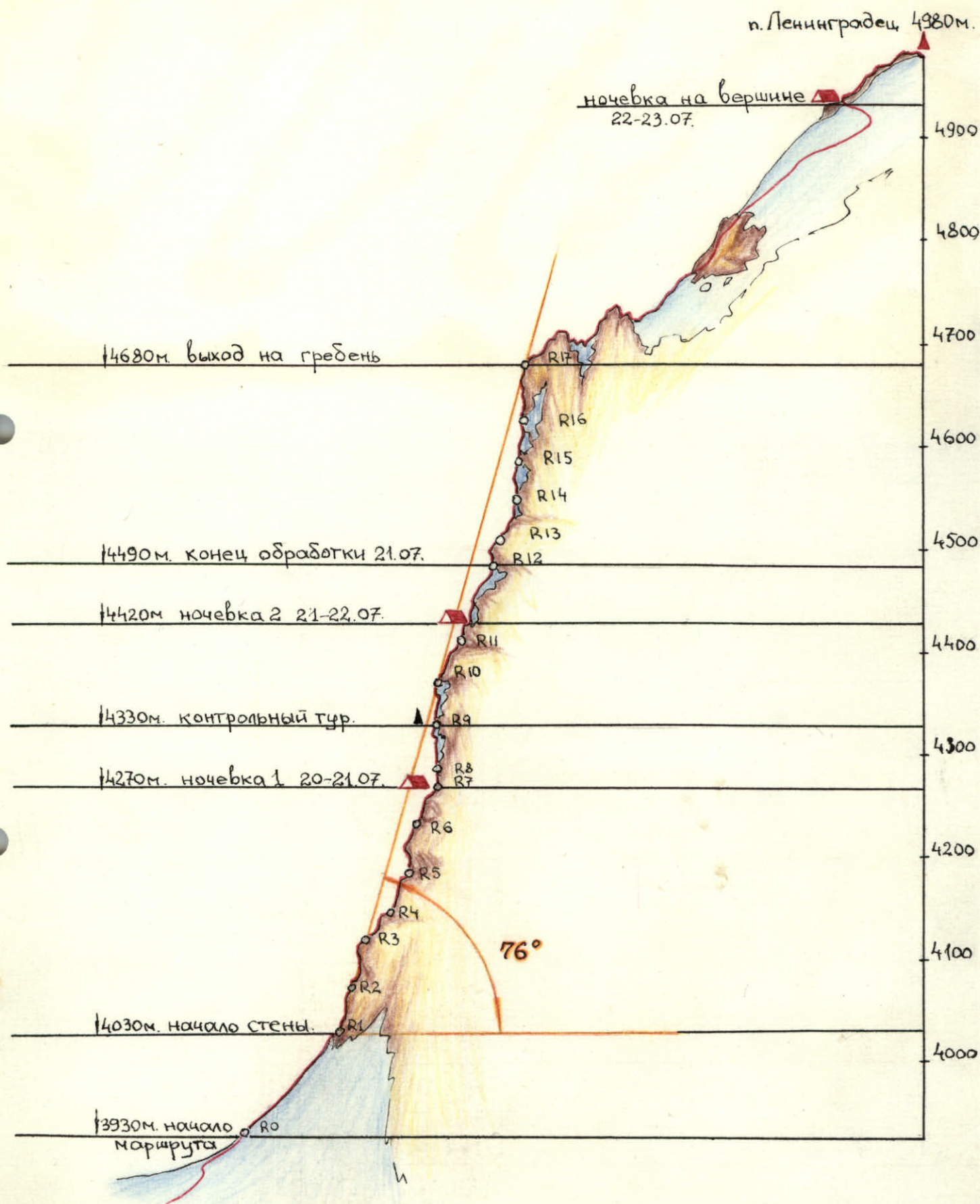
Рис. 2 Профиль маршрута. масштаб 1: 4000
